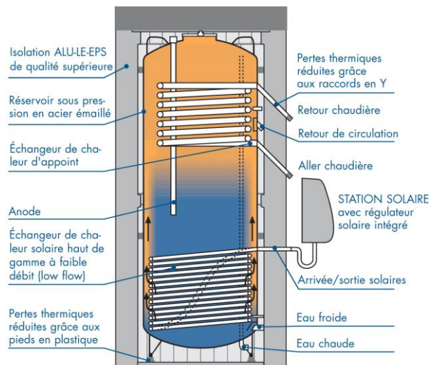
Coupe du COAX 390 (nouvelle version*)
